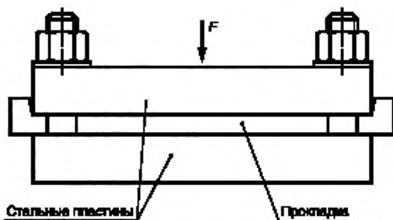
Рисунок 6 — Струбица для проведения испытаний
