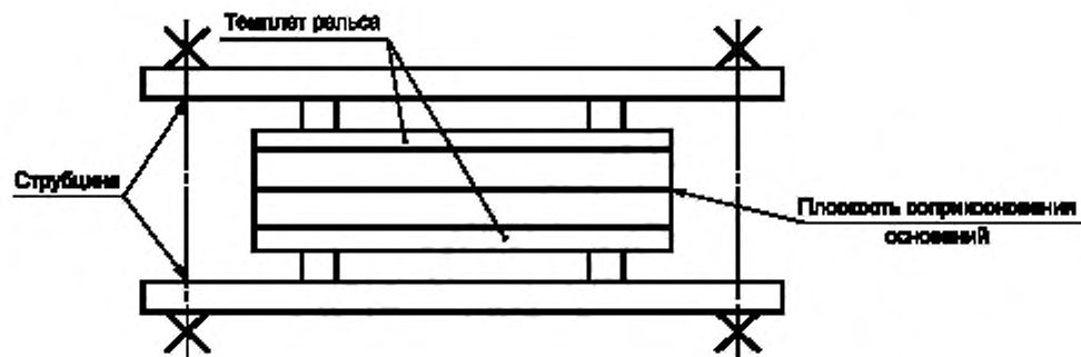
Рисунок 9 — Схема соединения двух тамплетов рельсов
